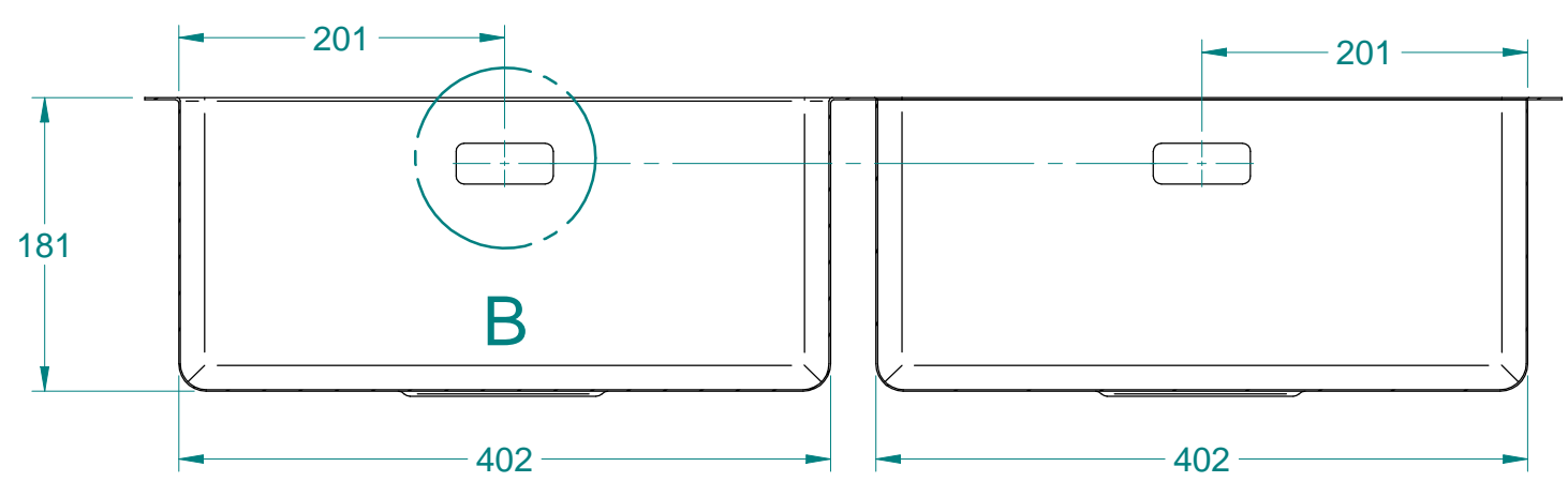
SECTION A-A
